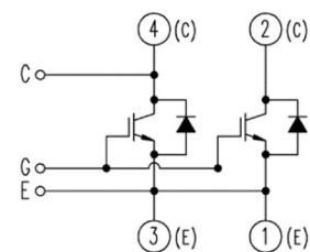
接線図 CIRCUIT DIAGRAM
